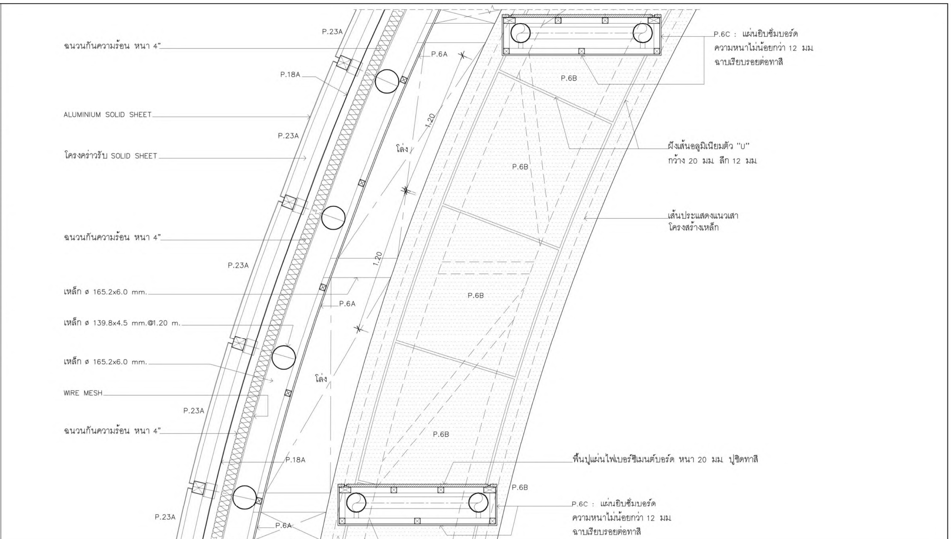
แบบขยาย 2 มาตราส่วน 1:20
