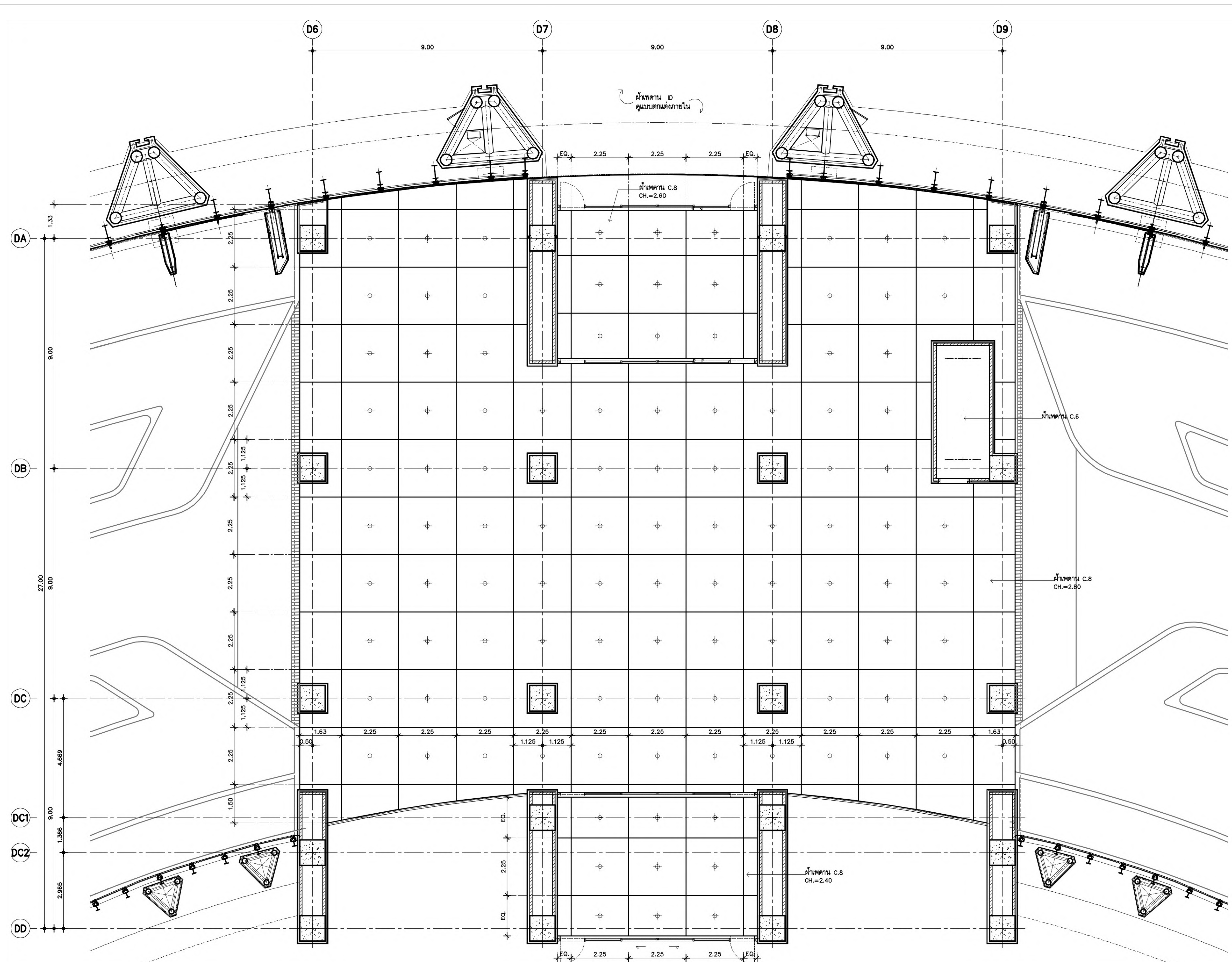
แปลนผ้าเพดานและดวงโคมโถงทางเข้า 2 มาตราส่วน 1: 75 ชั้นที่ 1 FFL+1.00
