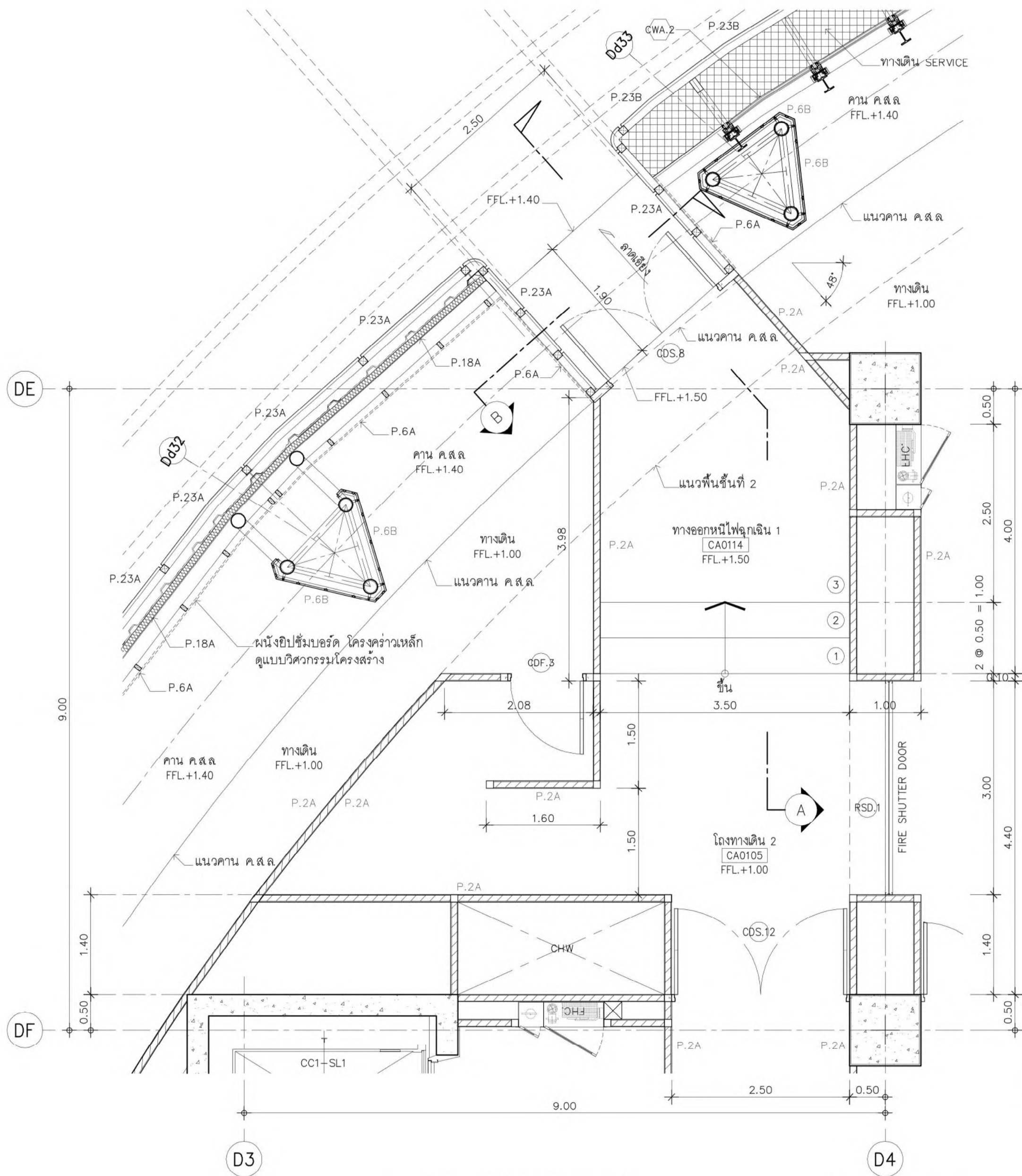
แปลนขยายทางหนีไฟ 1 มาตราส่วน 1:50 ชั้นที่ 1 FFL+1.00
