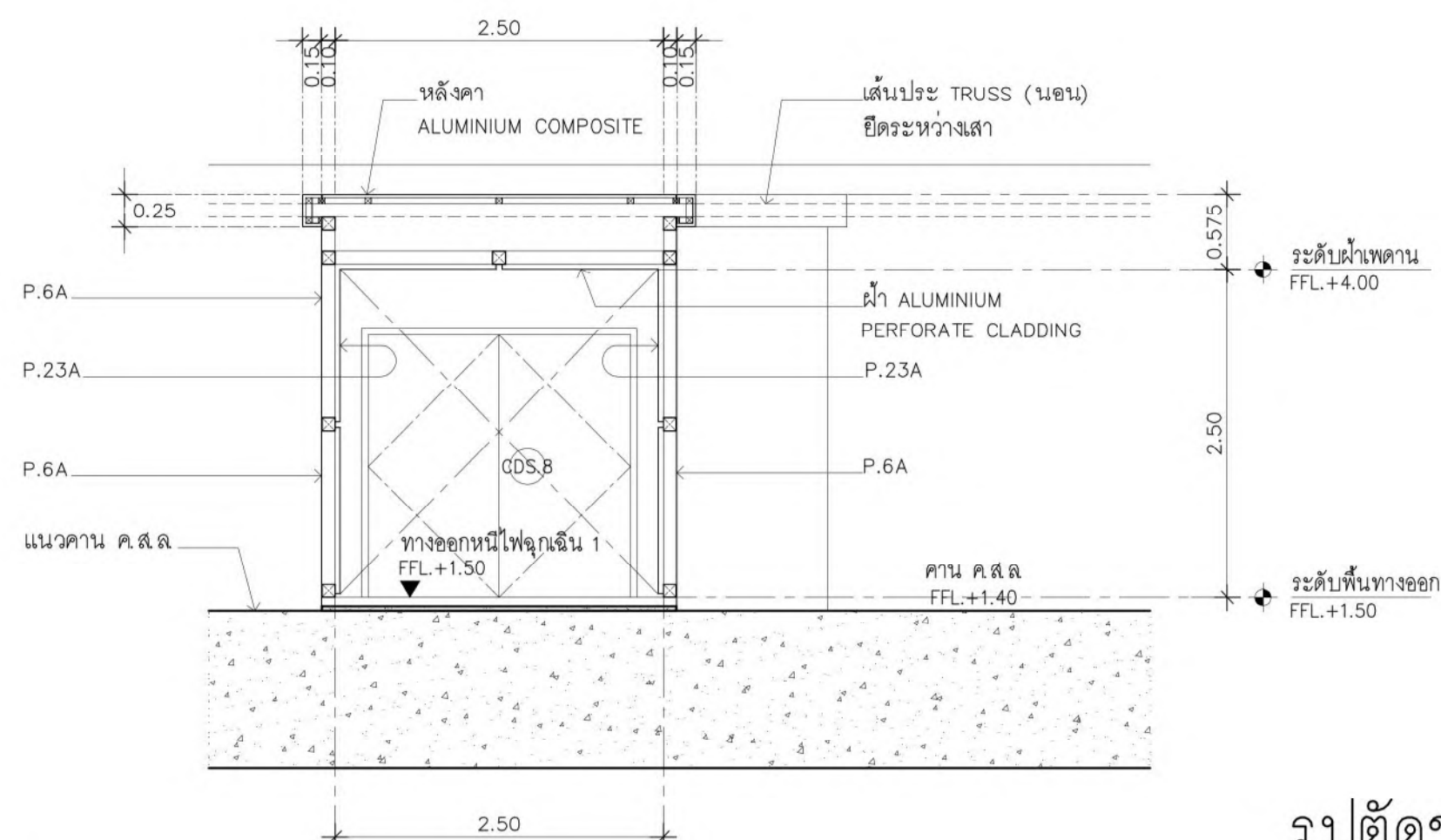
รูปตัดขยาย B มาตราส่วน 1:50
