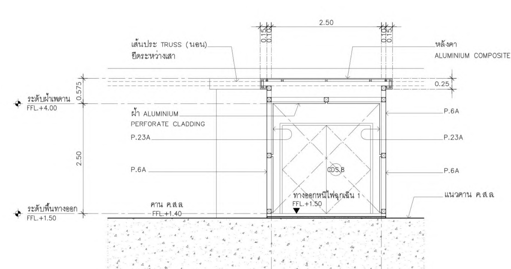
รูปตัดขยาย มาตราส่วน 1:50
