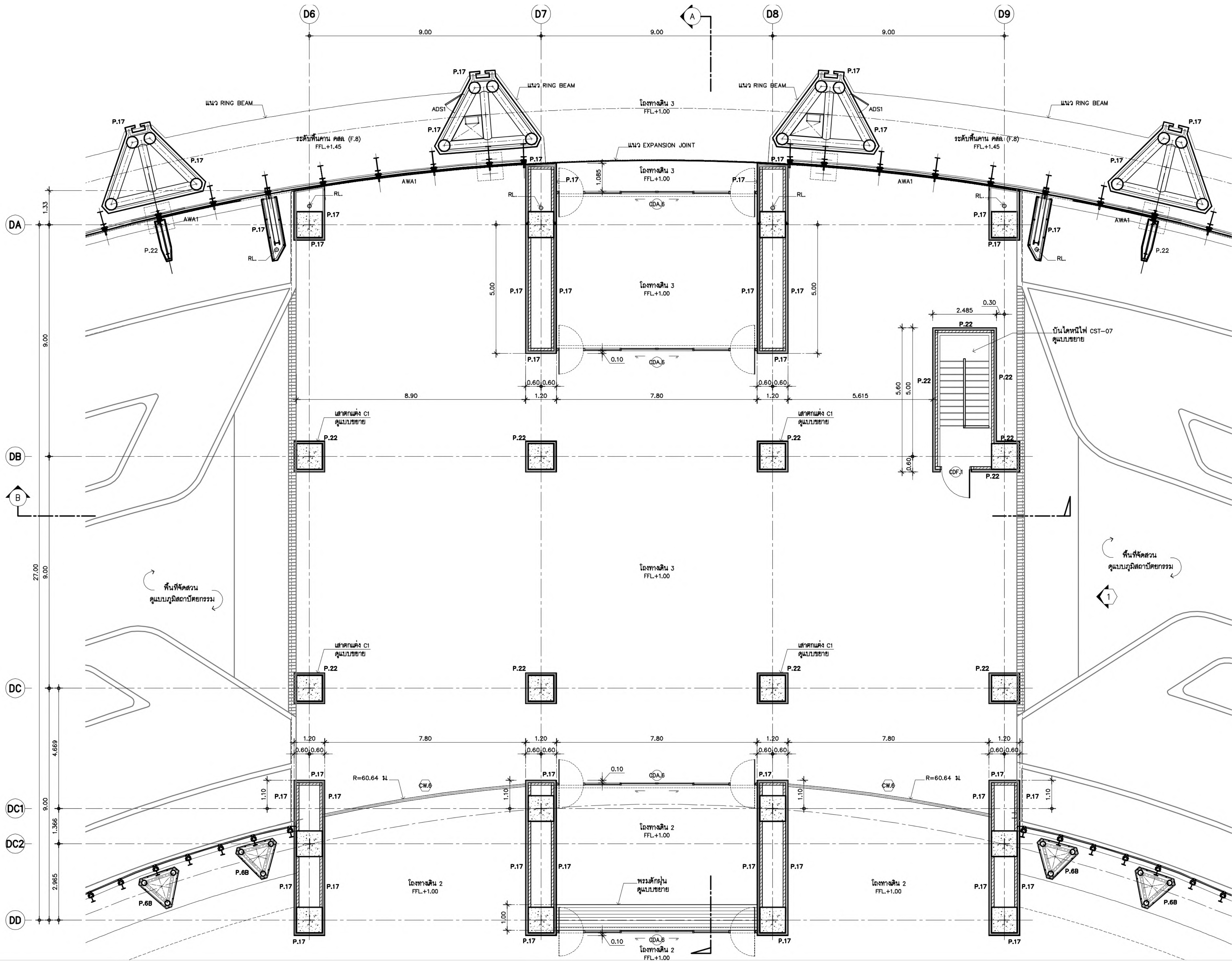
แปลนพื้นโครงสร้างเข้า 2 มาตราส่วน 1:75 ชั้นที่ 1 FFL+1.00
