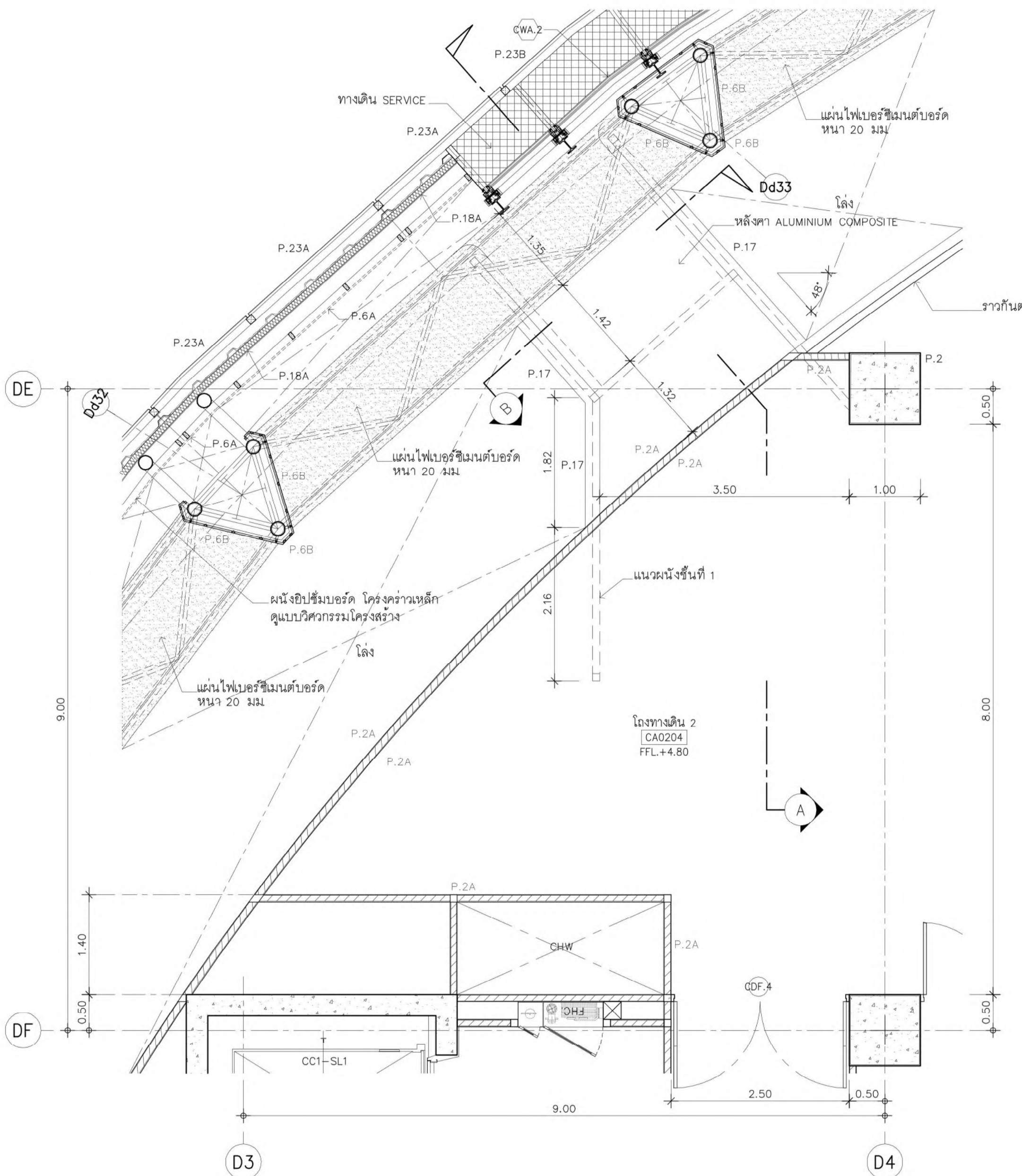
แปลนขยายทางหนีไฟ 1 มาตราส่วน 1:50 ชั้นที่ 2 FFL+4.80
