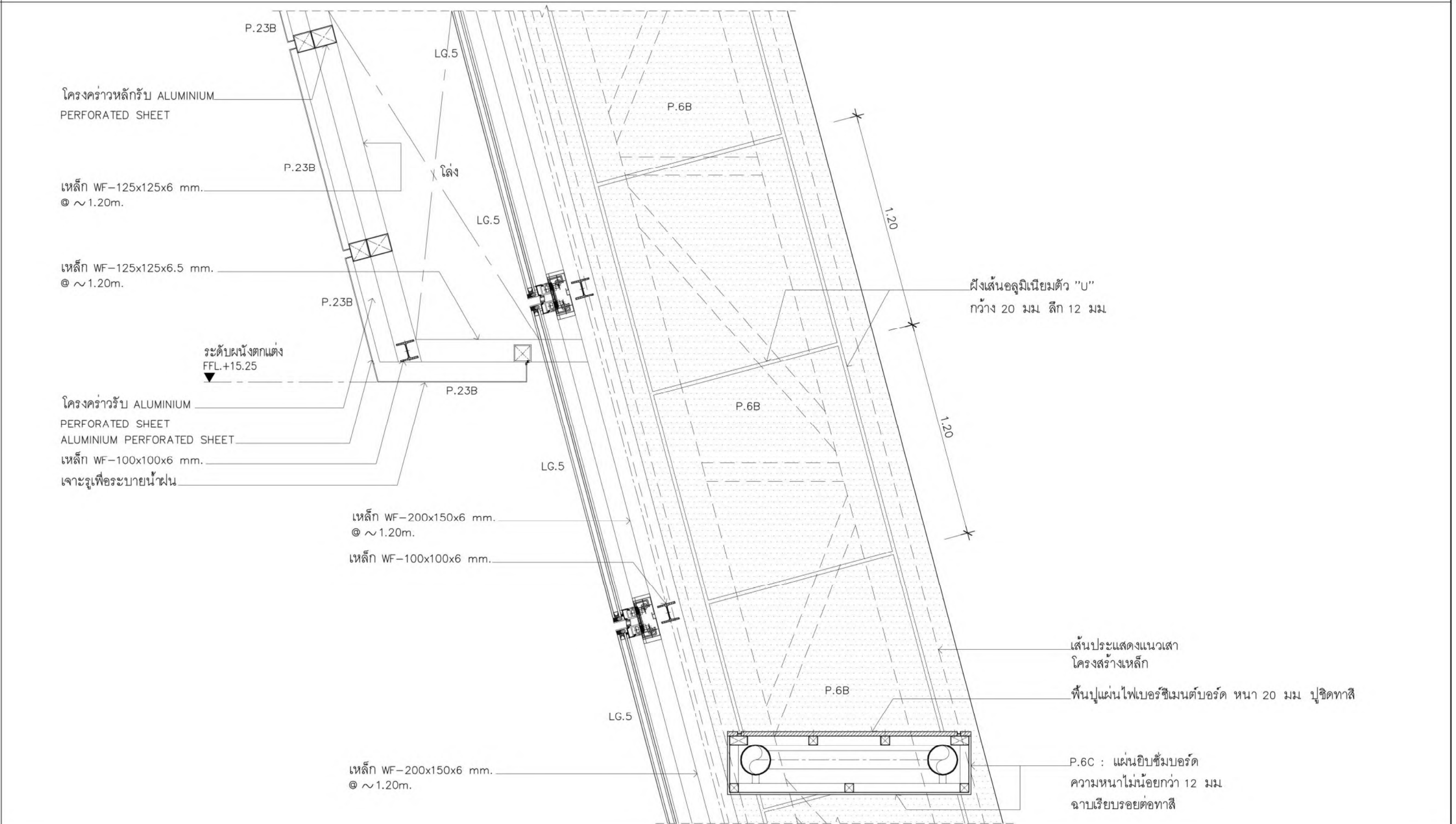
แบบขยาย มาตราส่วน 1:20
